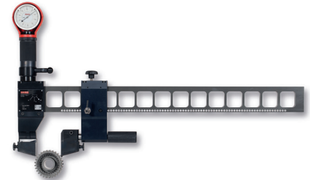
/ N7 - Zahnflankenprüfer
